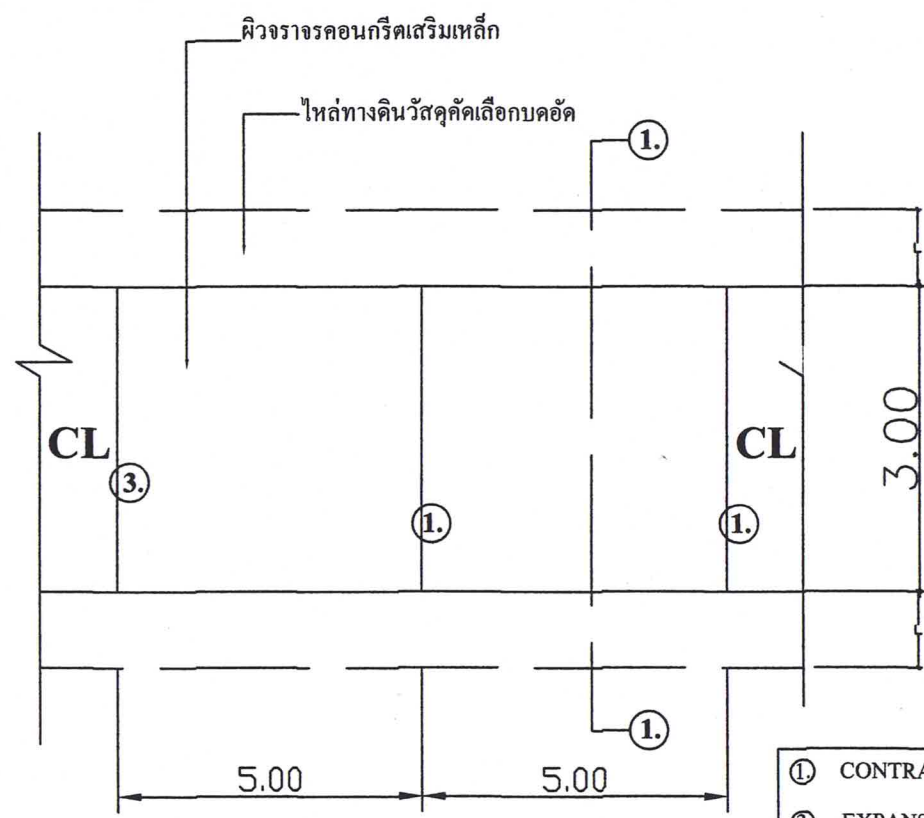
แปลนพื้น มาตรฐาน 1 : 75
